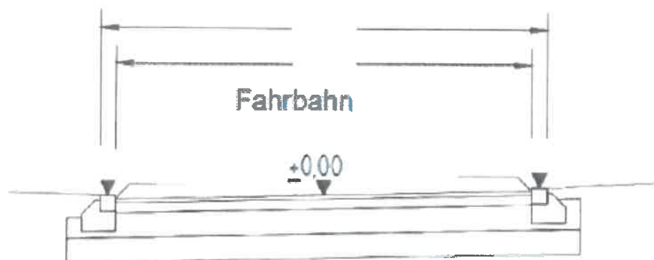
exemplarische Regelquerschnitte
